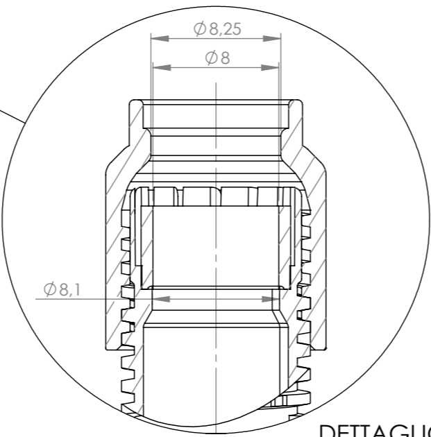
DETTAGLIO B SCALA 3:1
